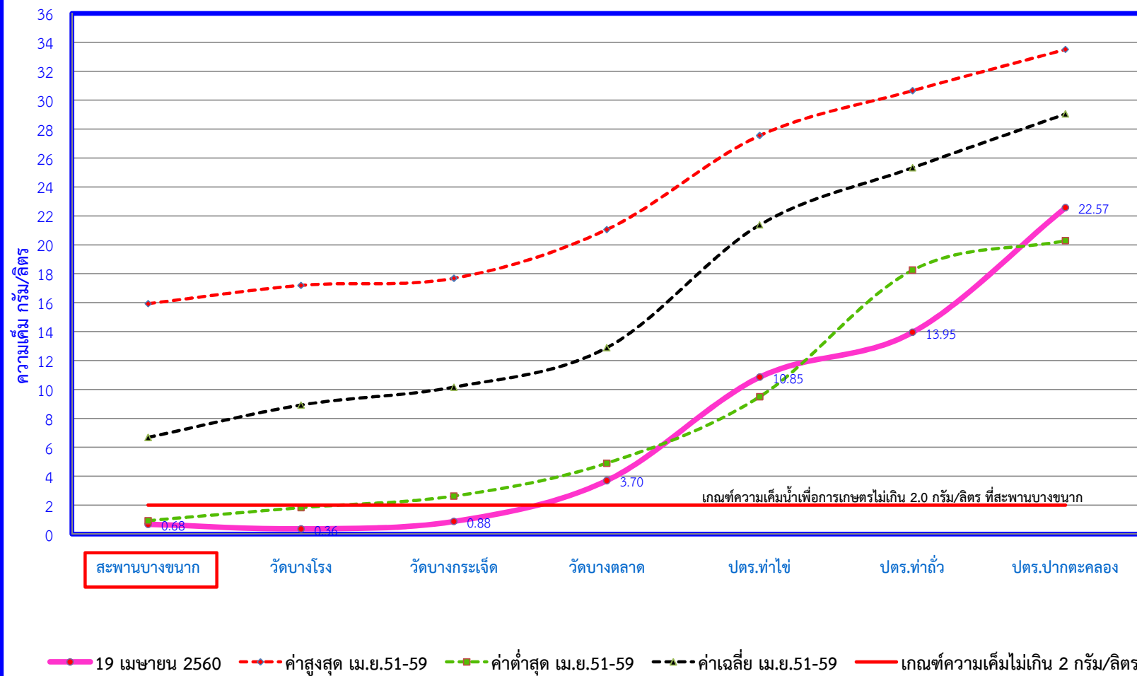
ค่าความเค็มในแม่น้ำบางปะกง วันที่ 19 เมษายน พ.ศ. 2560
